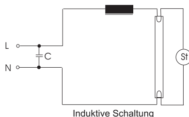
Induktive Schaltung
